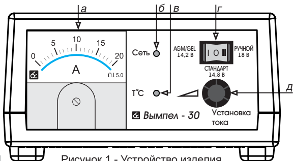
Рисунок 1 - Устройство изделия
